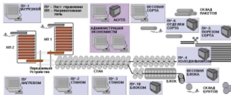
Рис. 1. Схема технологической линии сортопрокатного стана
